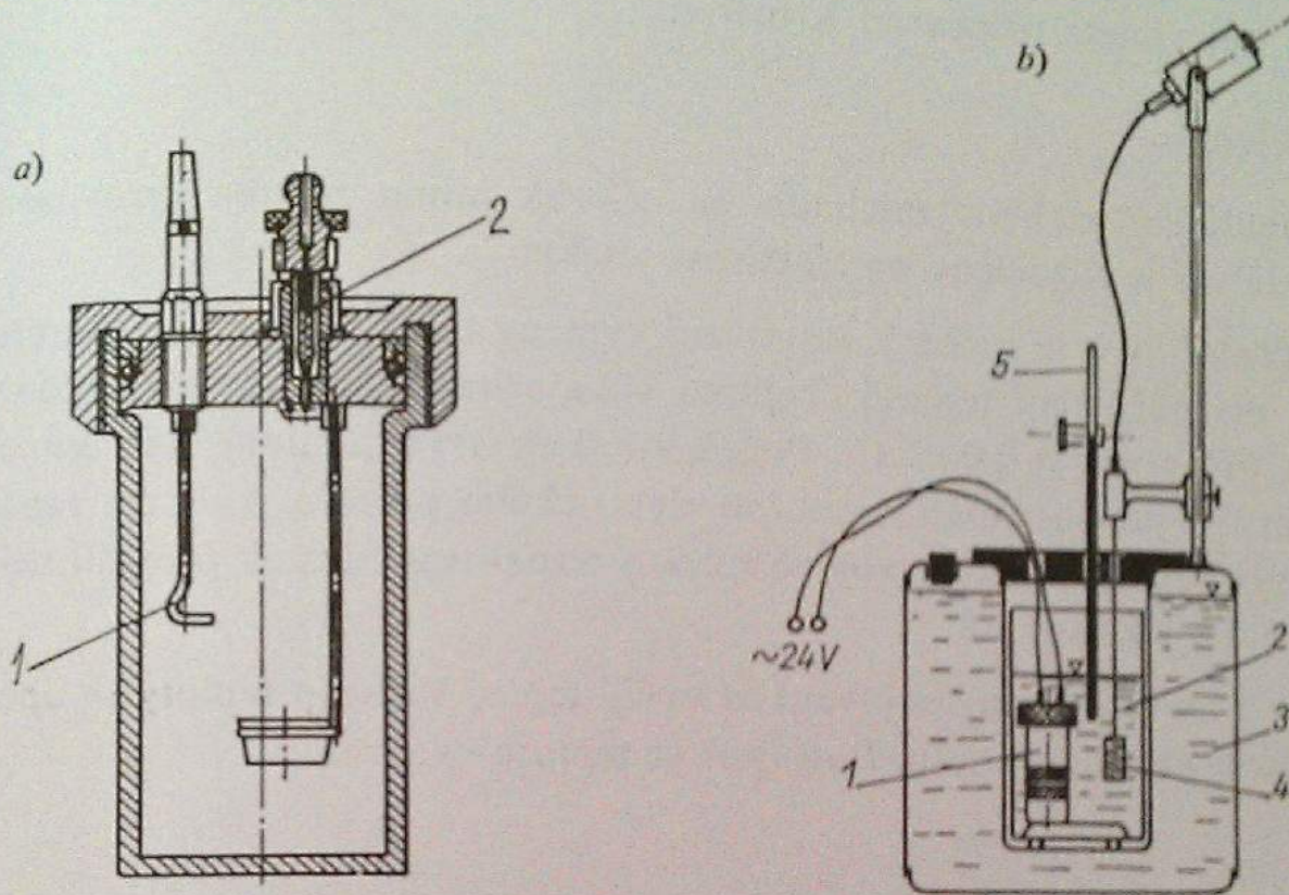
Obr. 280. Kalorimetr Karas - Šimek
